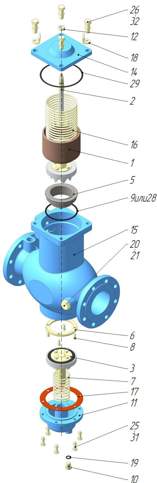
Рисунок В.2 – Клапан отсекающий 835.01.00.00
