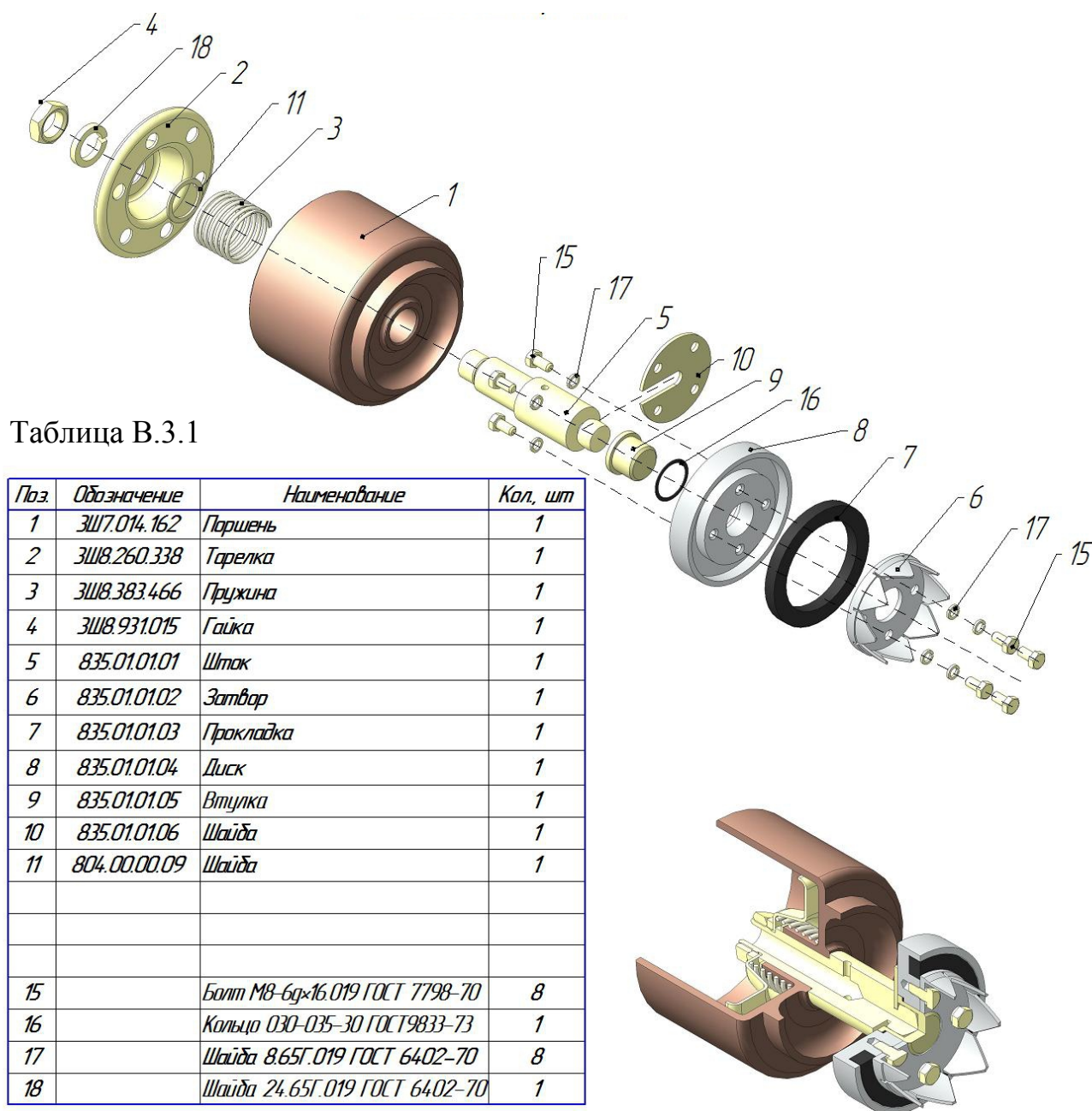
Рисунок В.3 – Поршень 835.01.01.00
