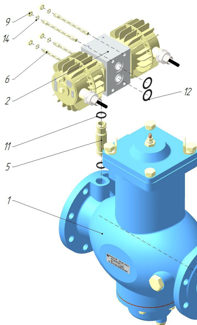
Рисунок В.1 – Клапан КО
