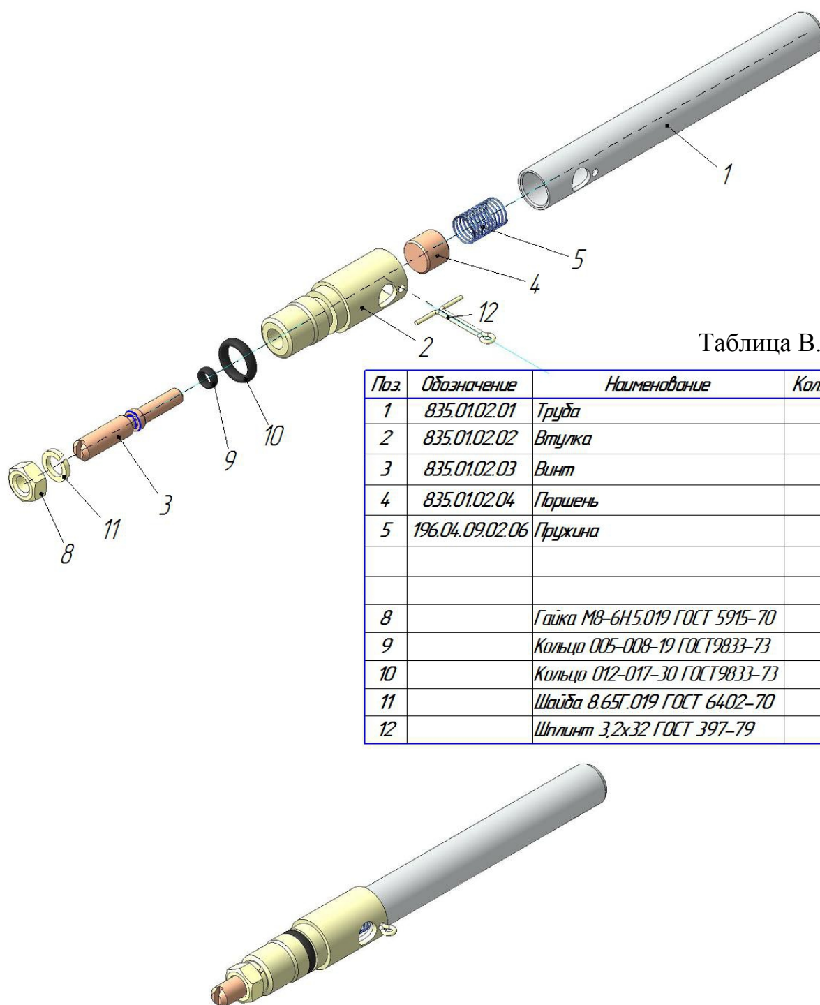
Рисунок В.4 – Регулятор 835.01.02.00
