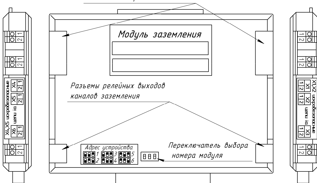
Разъемы подключения кабелей контроля заземления
