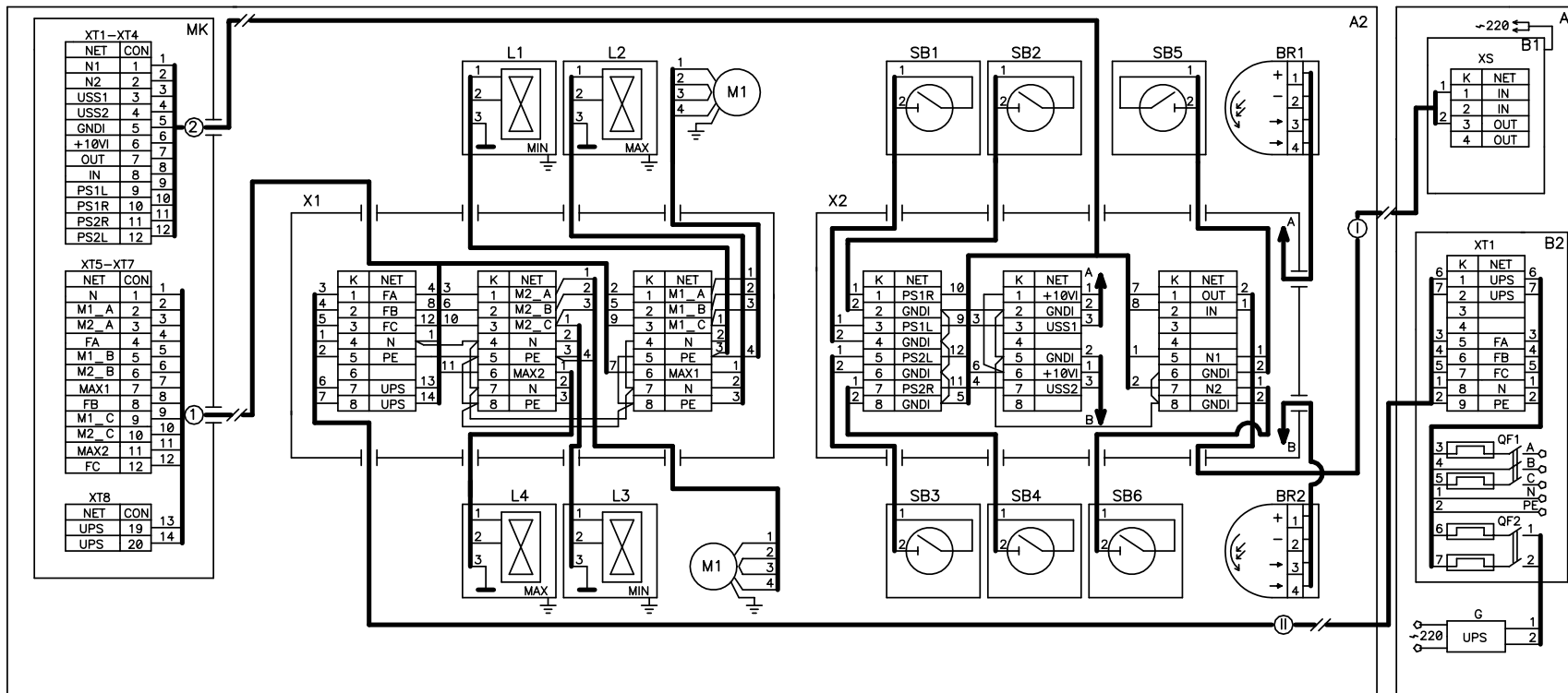
Рисунок А.1 Схема электрическая общая ТРК 2КЭД «Ливенка-22201», оснащенной контроллером КУП-1 (КУП-5).
