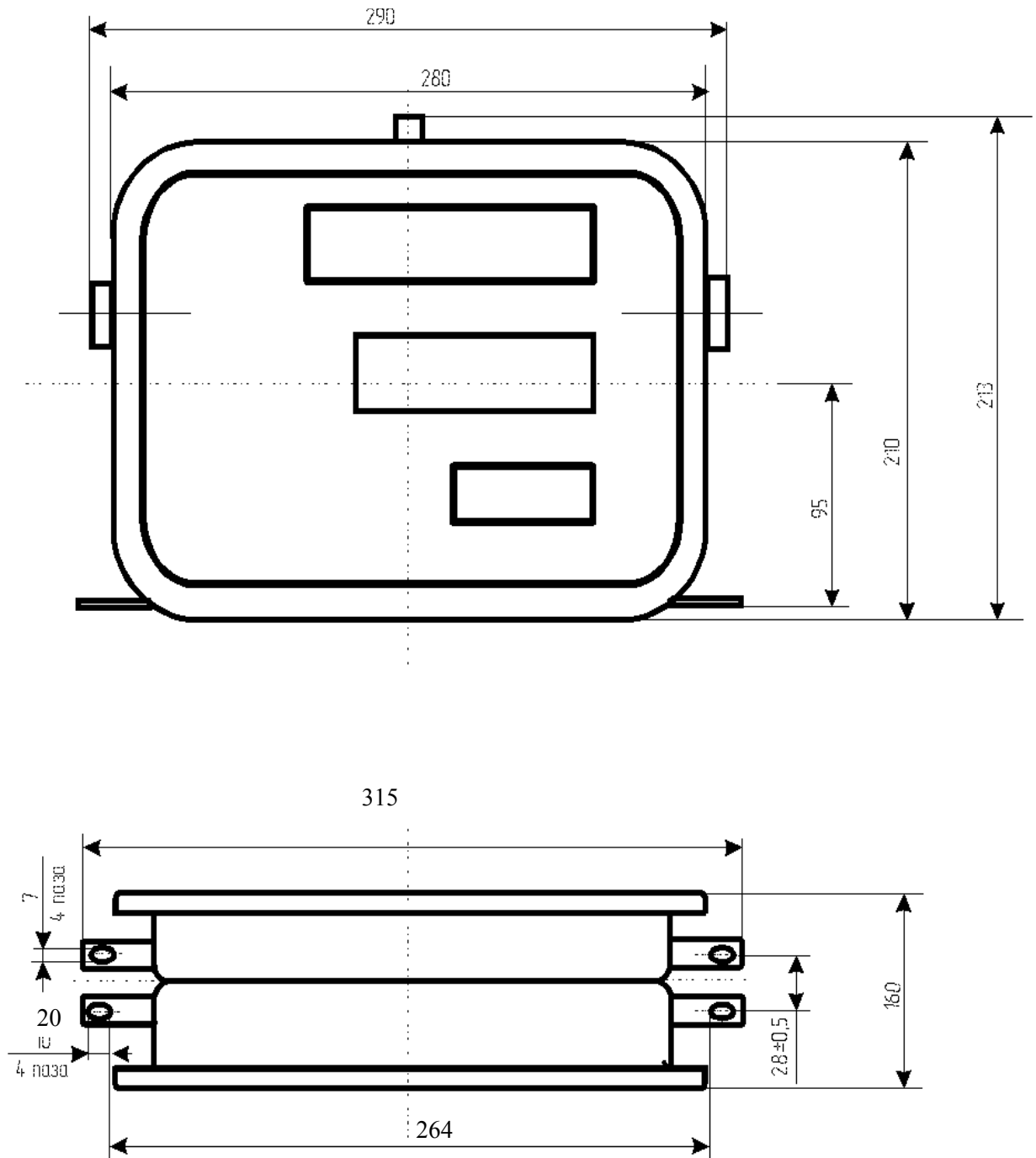
Рисунок Б.1 КУП-7, КУП-9. Габаритные и присоединительные размеры.
