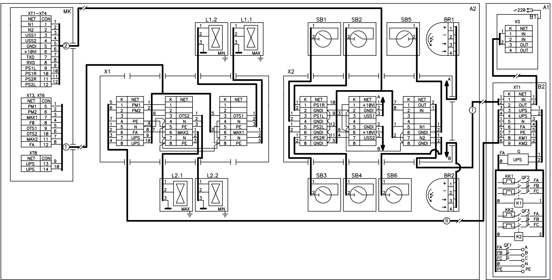
Рисунок А.1 Схема подключения ТРК 2КЭД «Ливенка-22200», оснащенной контроллером КУП-7 (КУП-9).
