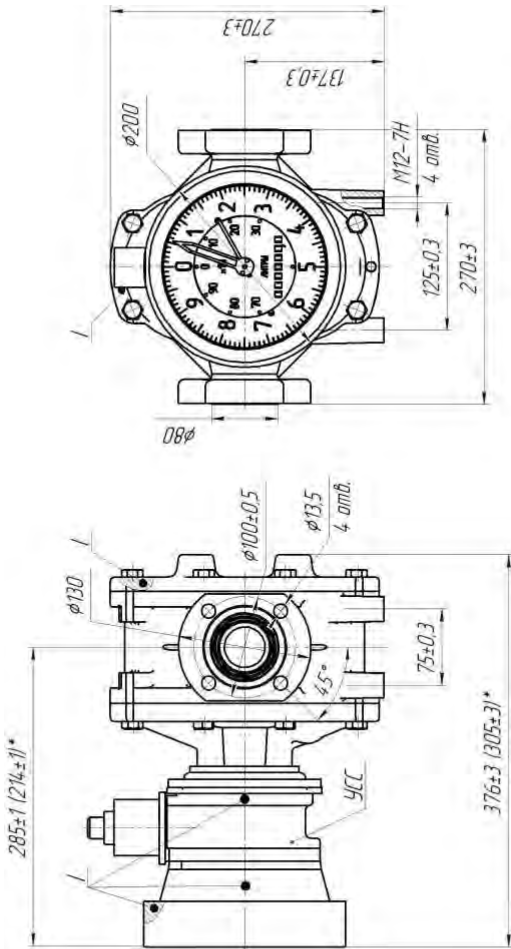
Рисунок Б.9 - Счётчик жидкости СЖ-ПШО-40-0,6-УСС Б-25-СУ;
